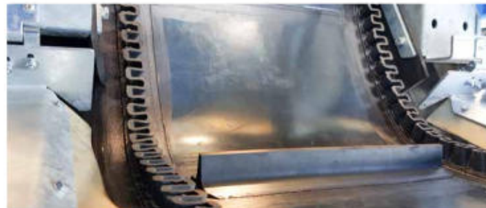
einteiliges Feinkornband
